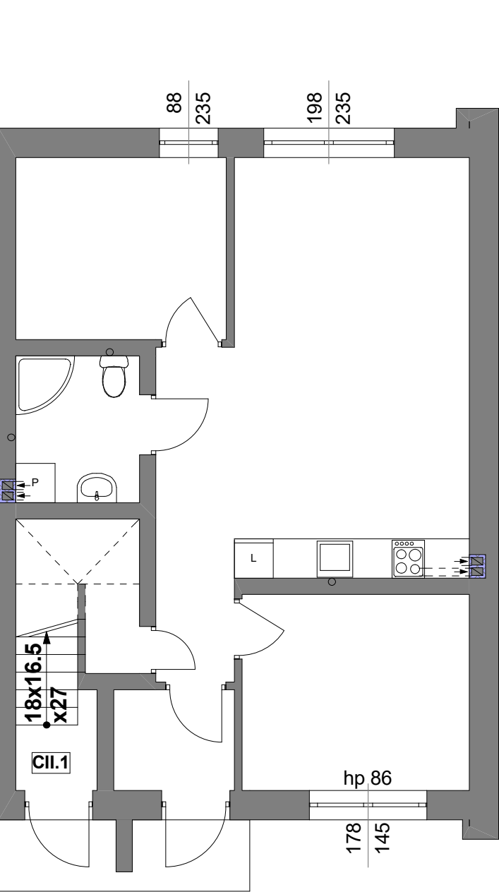
Budynek C- PARTER
