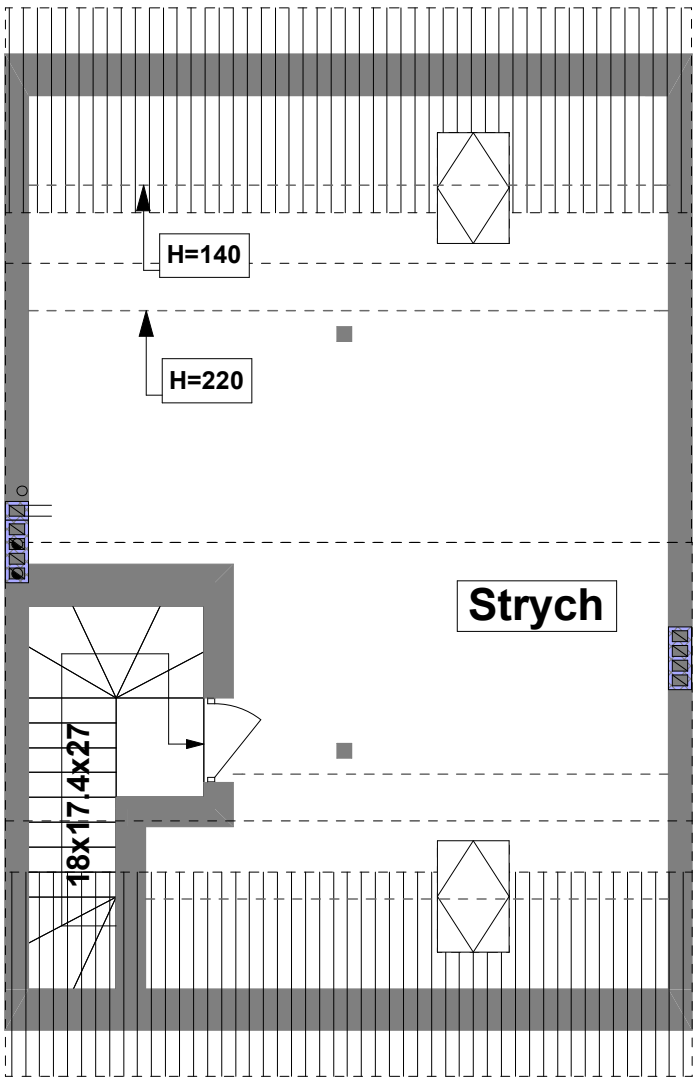
Budynek B- PODDASZE
