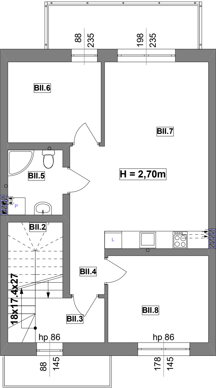
Budynek B- PIĘTRO
