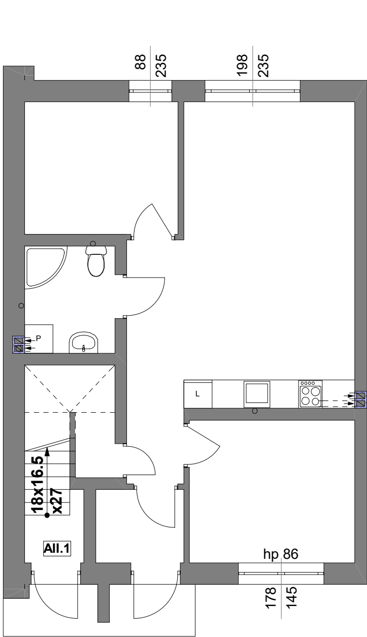
Budynek A- PARTER
