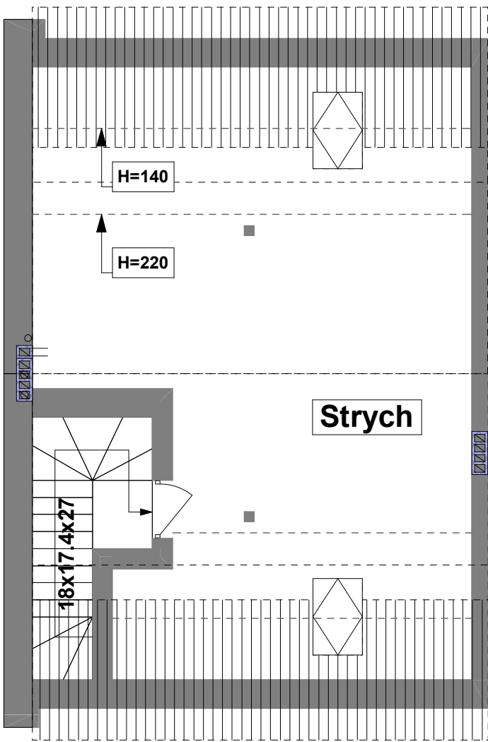
Budynek A- PODDASZE
