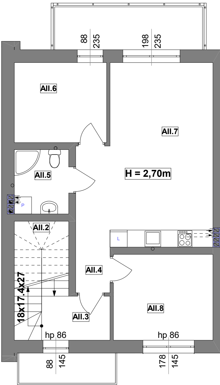
Budynek A- PIĘTRO
